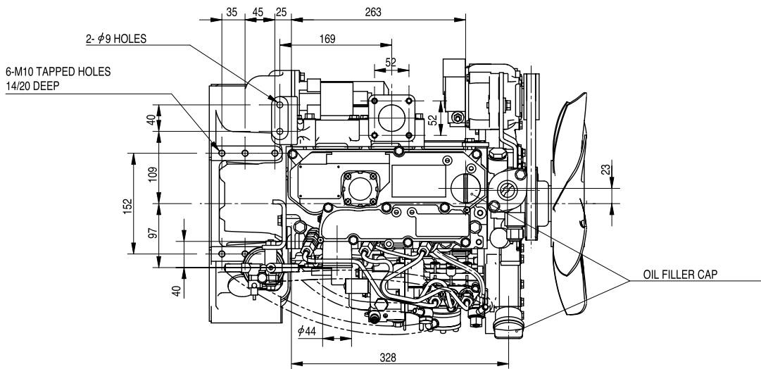
Top side
